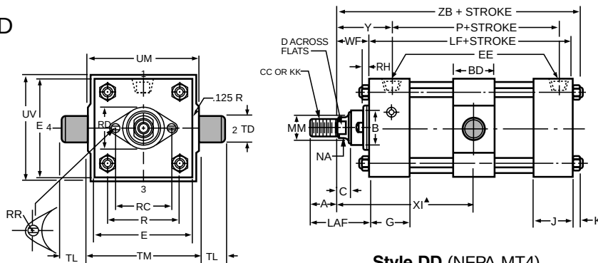
Style DD (NFPA MT4)
