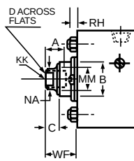
Style 9 Rod End (NFPA SF)
