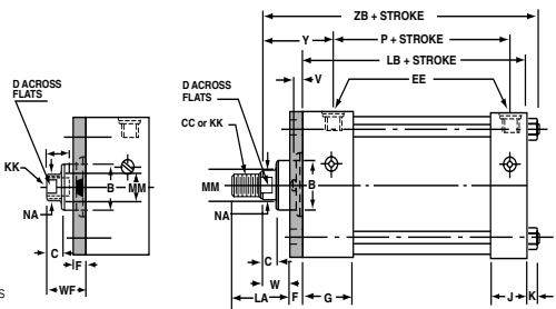
Style 9 Rod End (NFPA SF)
