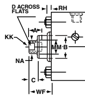
Parker Style 9 Rod End NFPA SF
