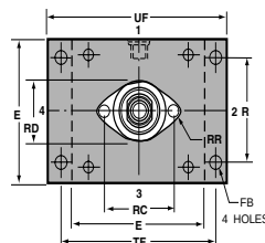
Style 9 Rod End (NFPA SF)
