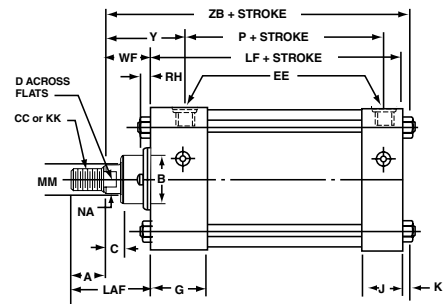
Parker Style 4 & 8 Rod End NFPA SM & IM
